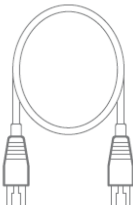
Netzwerkkabel
