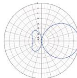
Vertikal | 390MHz
