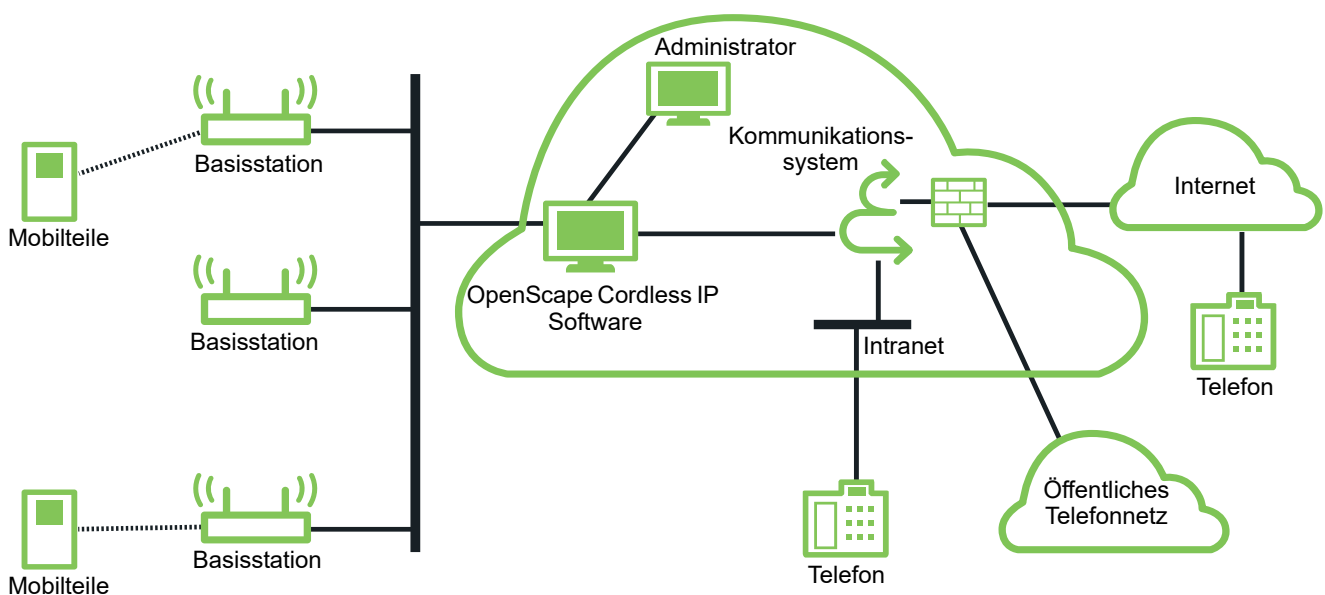
Konfiguration/Systemkonzept
