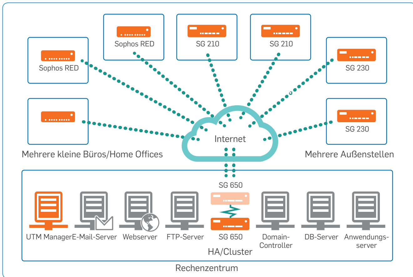
Bereitstellungsszenario mit einem Cluster aus zwei SG 650 Appliances als Teil eines weitverzweigten Großunternehmens mit Sophos REDs zum Schutz von kleinen Büros und Home Offices sowie weiteren SG Appliances zum Schutz von Außenstellen
