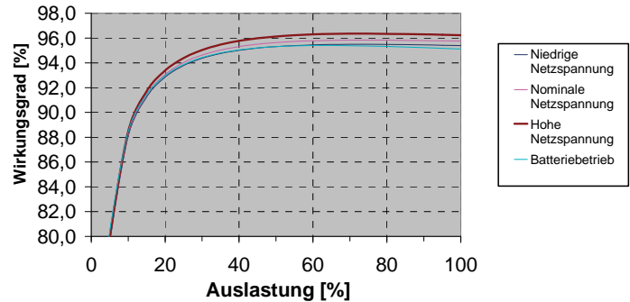
Galaxy 3500 30kVA Wirkungsgrad
